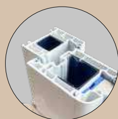
DORMANT 67x70MM & OUVRANT 105x70MM RENFORCÉS
