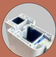
DORMANT 67x70MM & OUVRANT 105x70MM RENFORCÉS
