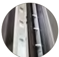
BARRE ANTI-DÉGONDAGE EURASTOP Barre en acier 12 pions anti-dégondage sur toute la hauteur de la porte. En option.
